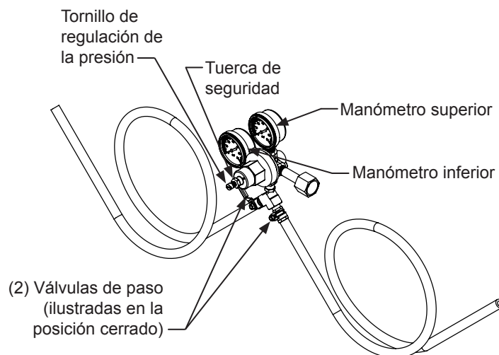
Figura 40 (Regulador de torre para dispensado doble)
